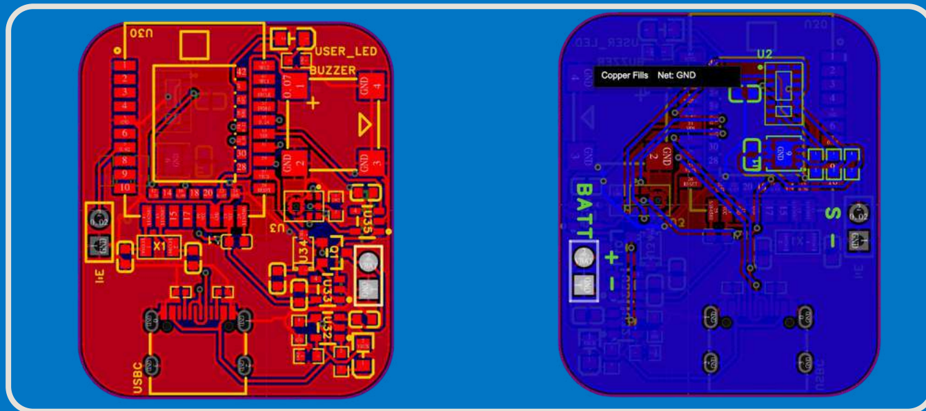
Собранная печатная плата (лицевая/обратная сторона)
